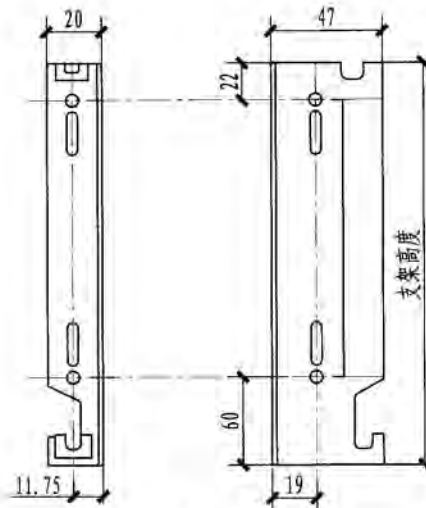
普通支架
