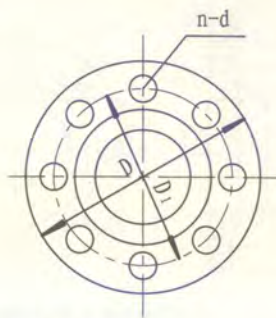
可曲挠橡胶接头详图
