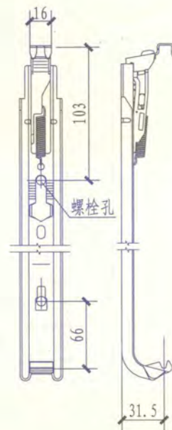
弹簧支架
