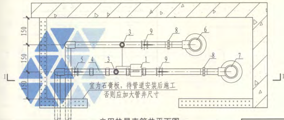
户用热量表管井平面图
