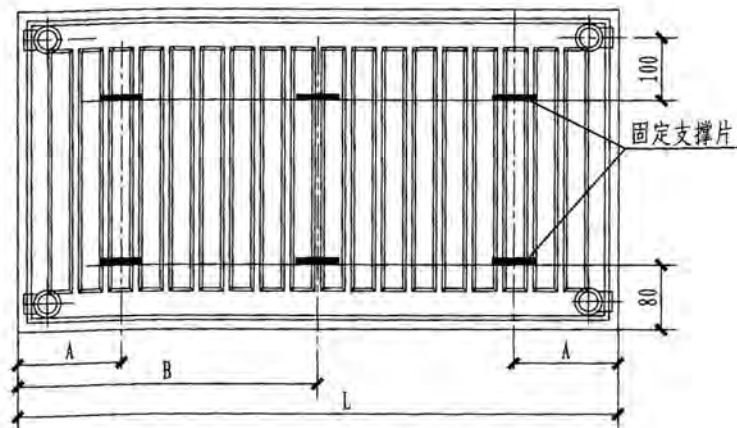
散热器固定片设置位置示意图
