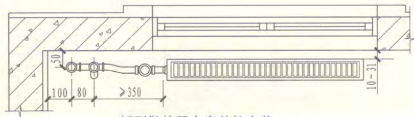
板型散热器在窗前的安装
