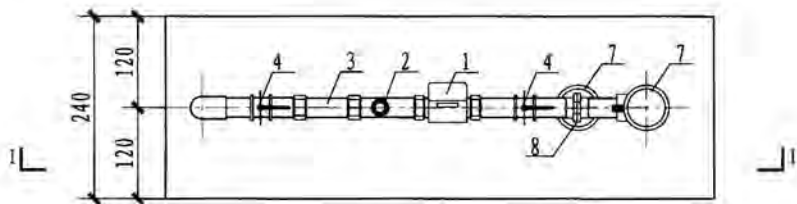
户用热量表箱平面图
