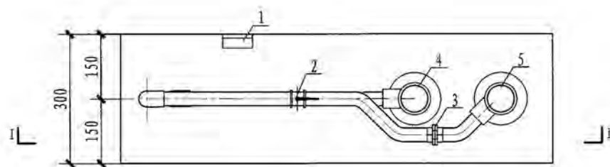
户用热量表箱平面图
