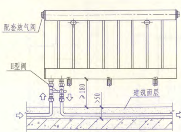
地面敷设单管系统散热器连接 (二)
