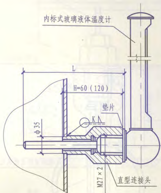
90°角型温度计安装图
