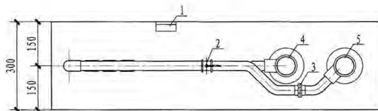
户用热量表箱平面图
