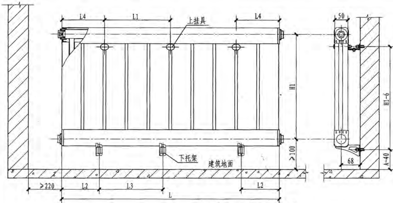
铜铝复合柱翼型散热器的安装
