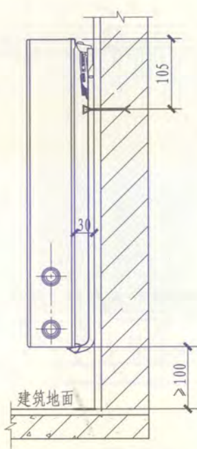
S、Dp系列 弹簧支架挂墙安装
