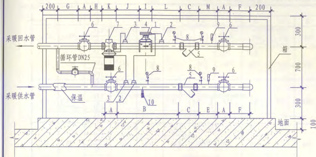
I-I 剖面
