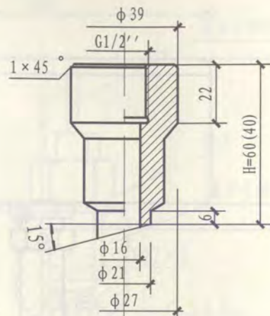
15°角接头
