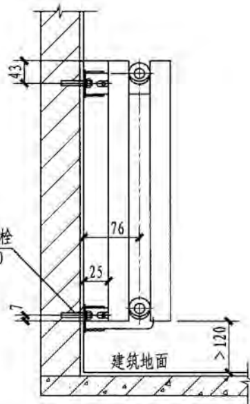
双排D型管与圆管焊接 散热器挂墙安装
