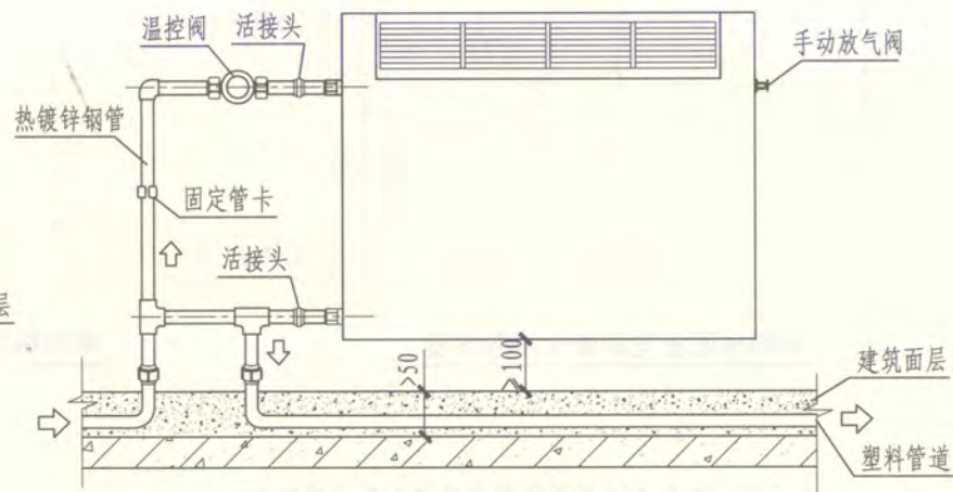
地面敷设单管系统散热器连接
