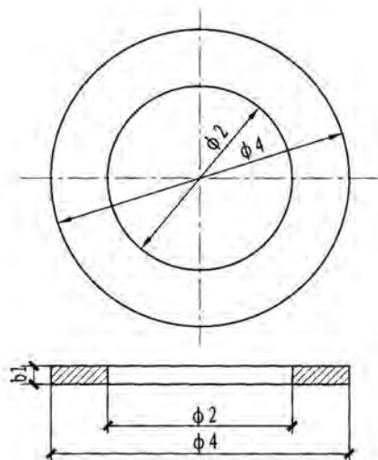
翼 环
