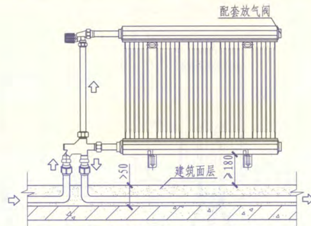
地面敷设单管系统散热器连接 (三)
