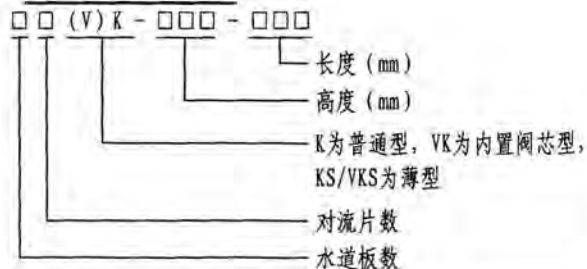
散热器型号标记:
