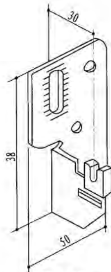
德式支架
