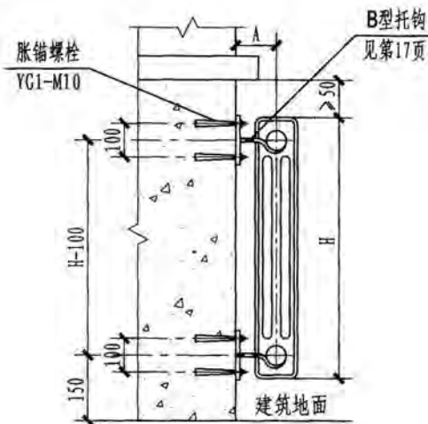
混凝土墙上安装(II)
