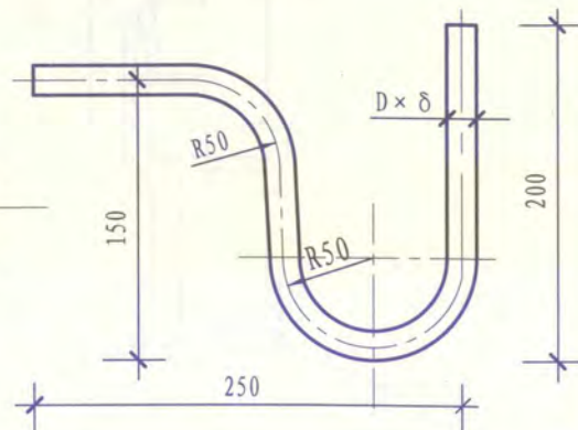
冷 凝 弯
