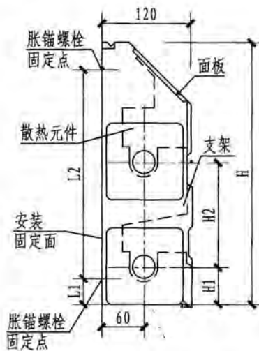
CB系列B型散热器
