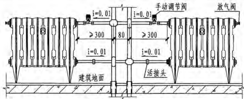
双管散热器双侧连接
