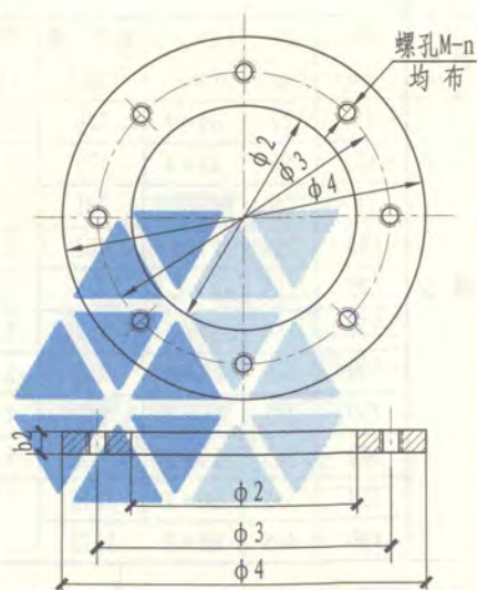
翼盘
