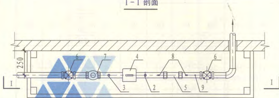
I-I 剖面
