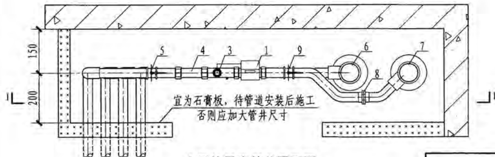
户用热量表管井平面图
