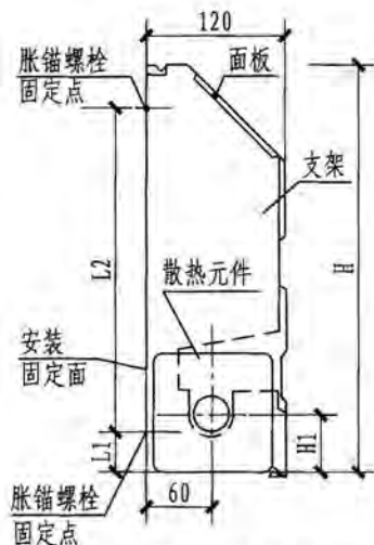
CB系列A型散热器
