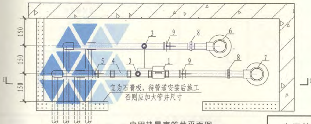
户用热量表管井平面图
