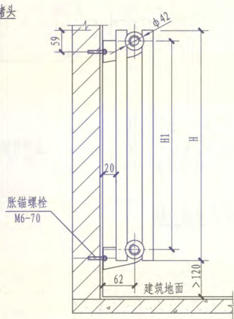
双排椭圆管与圆管焊接散热器挂墙安装
