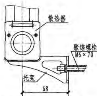
铜管铝翼散热器下托架详图
