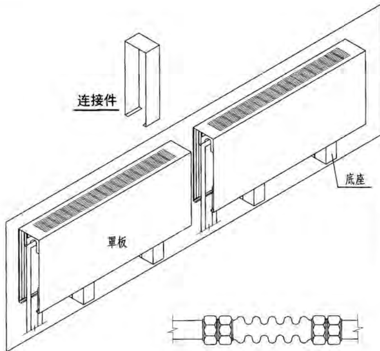
按需要设置软连接
