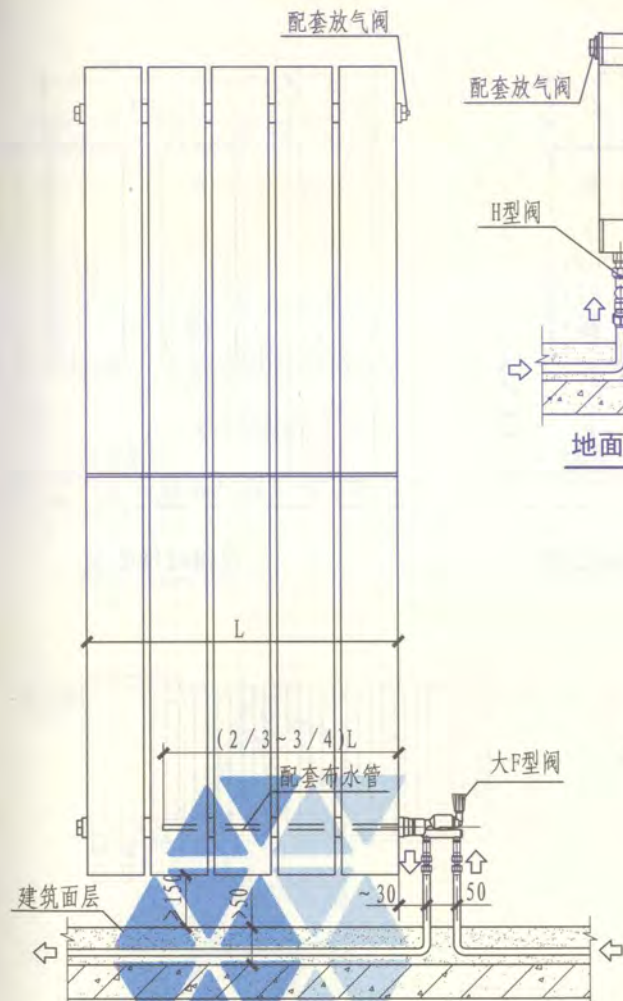
地面敷设单管系统散热器连接 (一)
