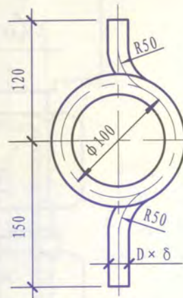
冷 凝 圈
