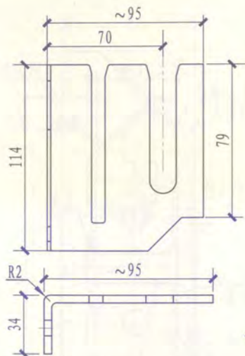
单排散热器固定托架
