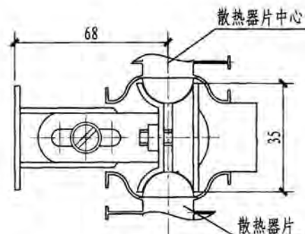
散热器上挂具安装俯视图
