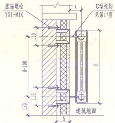
保温复合墙上安装 (III)
