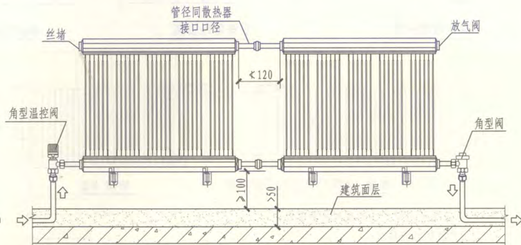
地面敷设双管系统散热器连接
