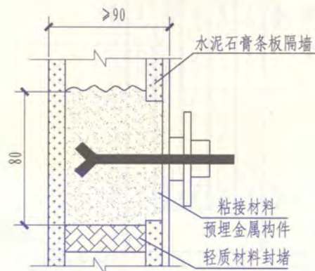
水泥、石膏条板预埋件节点
