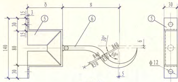
C型托钩
