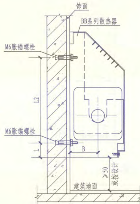
BB系列散热器单体挂墙安装
