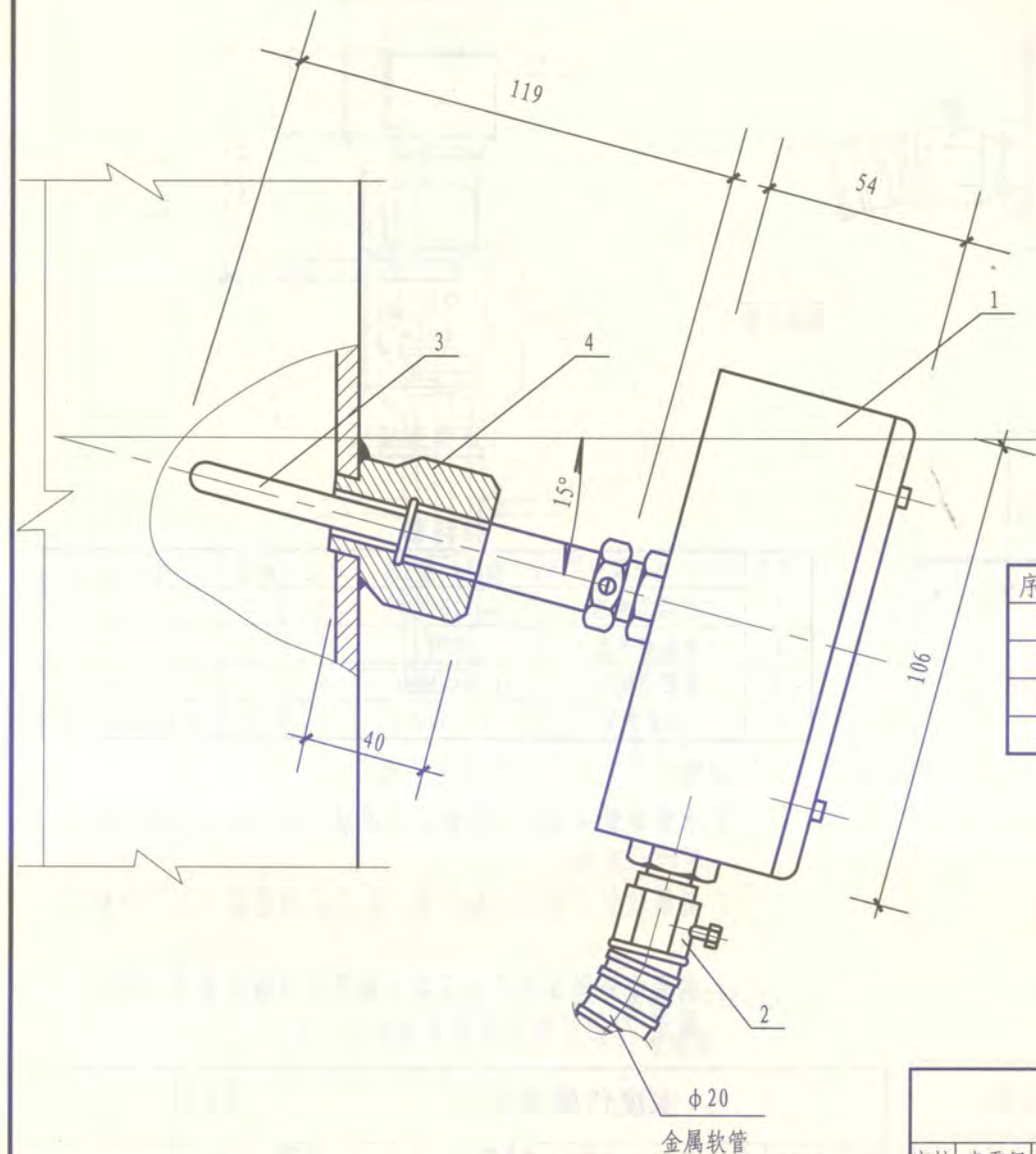
温度传感器安装
