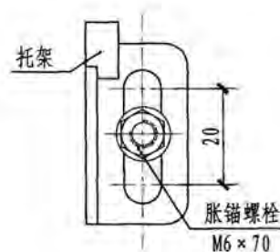
散热器下托架安装图
