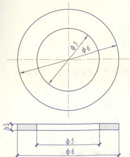
挡圈
